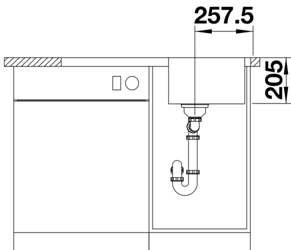
Frontansicht
