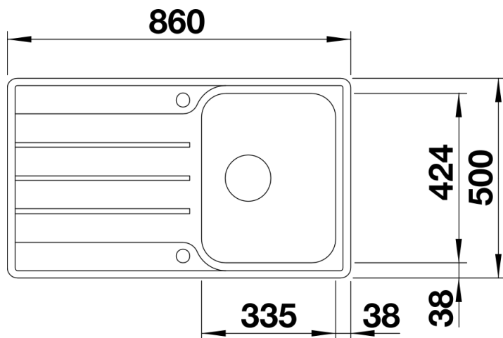
Aufsicht
