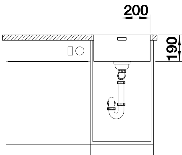
Frontansicht
