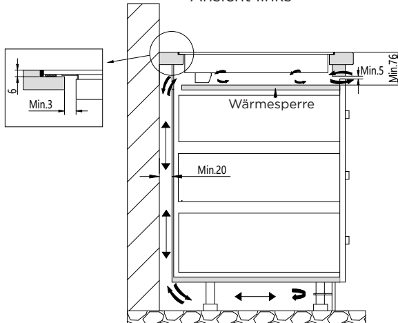
Ansicht links
