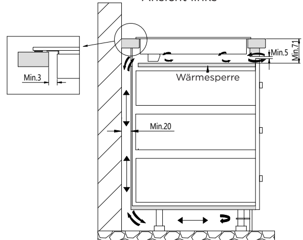
Ansicht links
